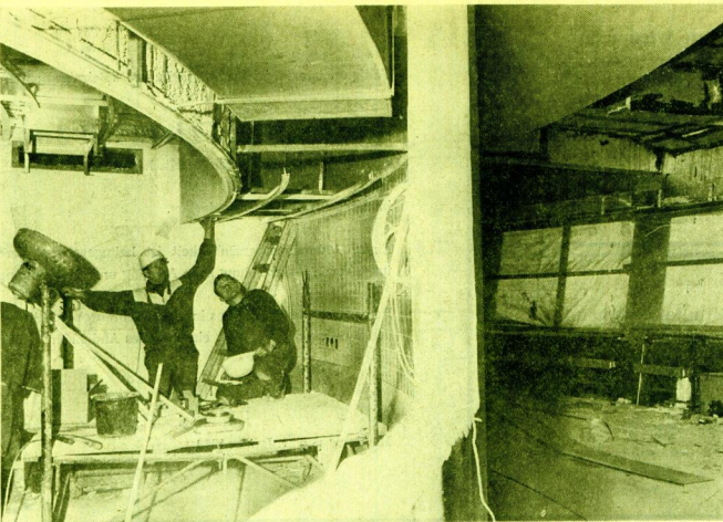
In 128 Meter Höhe: links die Küche, rechts das Drehrestaurant. Rechts unten der Spalt zur Drehscheibe. Fotos: Mihaly Malyday
