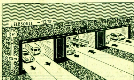
Der Querschnitt des neuen Elbtunnels. Sechs Fahrpläne in drei Röhren.
